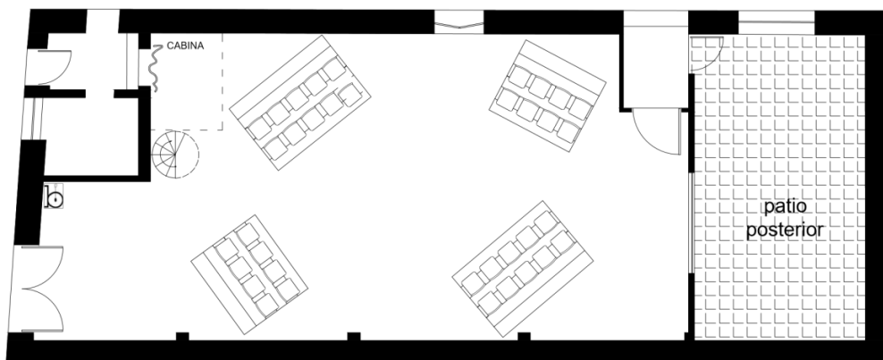
PLANO ARQUITECTONICO
